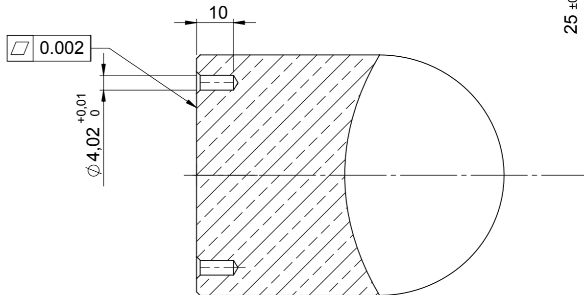
SCHNITTDARSTELLUNG B-B
